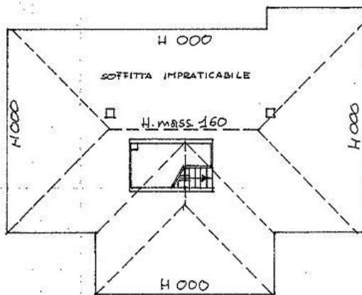
PIANTA SOTTOTETTO
